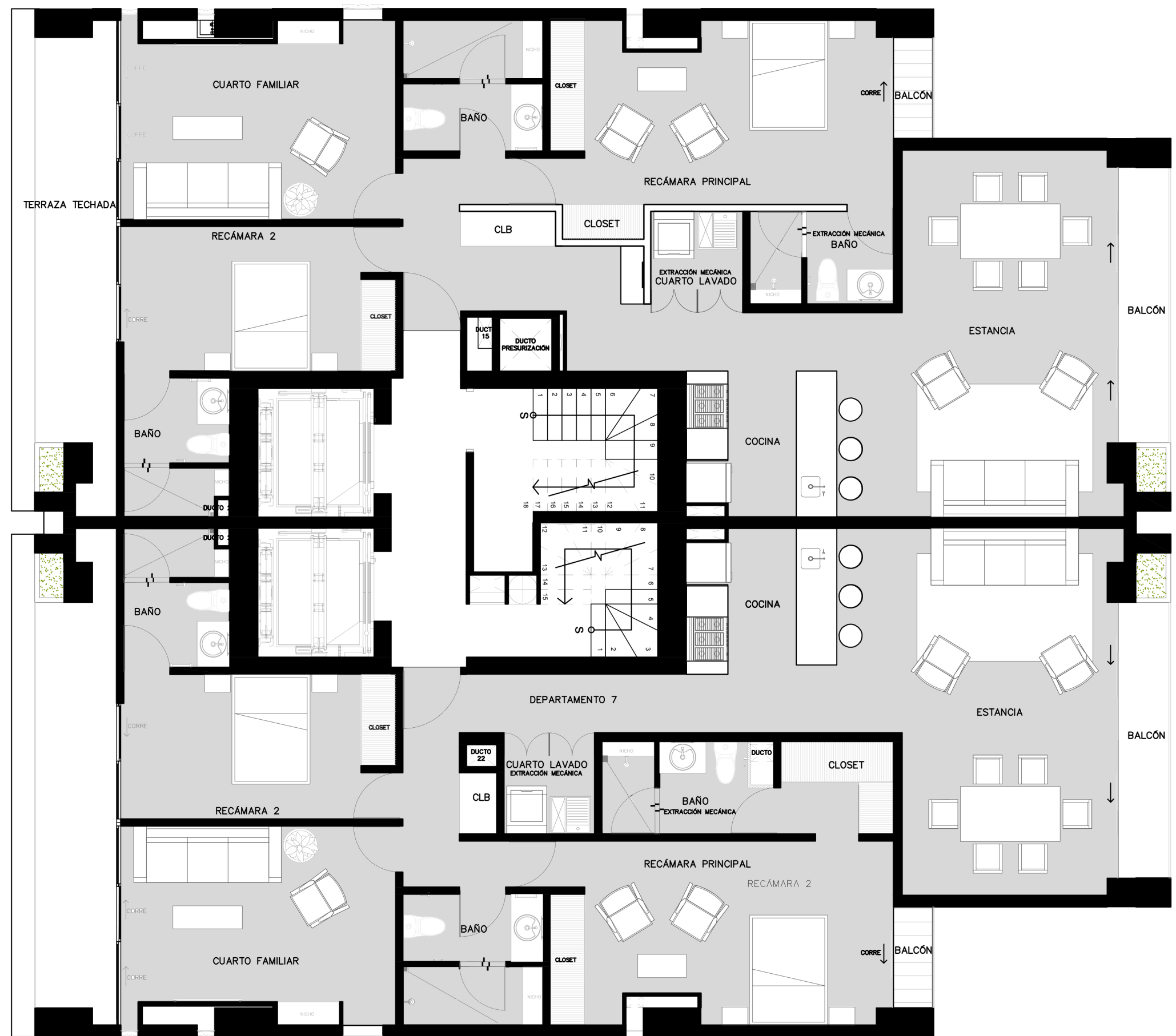
TIPO DEPARTAMENTOS N26
